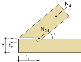
Ferserversatz (F)
