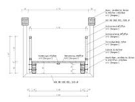
Querschnitt M 1:25
