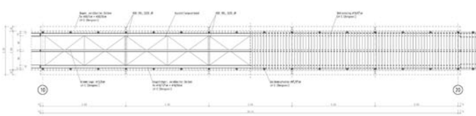
Draufsicht M 1:50
